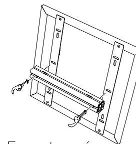
Format carré 480x480 mm
