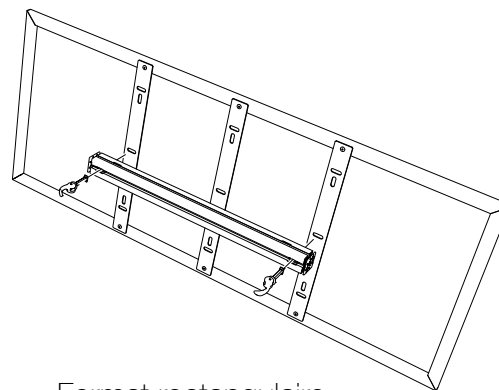
Format rectangulaire horizontal 1200x480 mm
